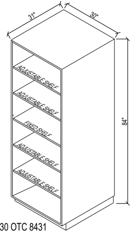
30 OTC 8431
