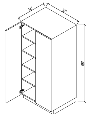
30 TC6524
