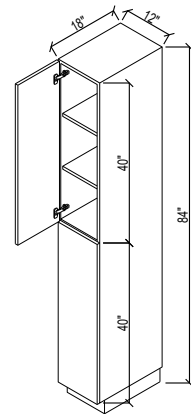
12 TC 8418 H
